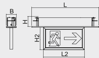
Deckeneinbau
