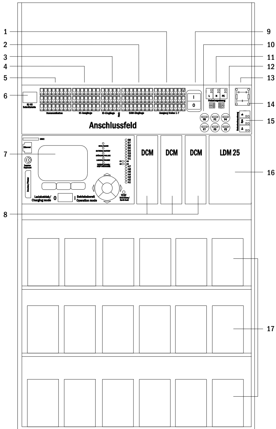
Abbildung 1: Innenansicht
