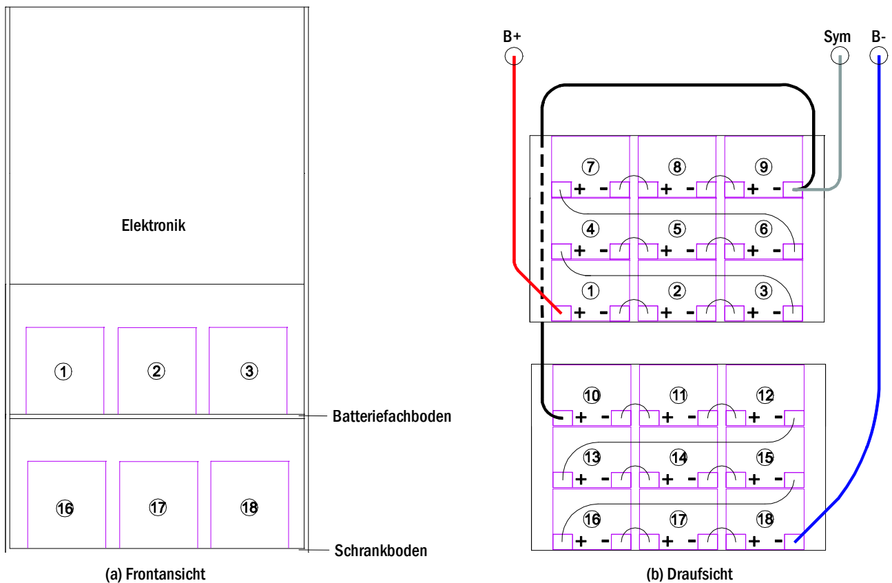
Abbildung 14: Aufstellung und Verschaltung der Batterieblöcke 12V 5Ah
