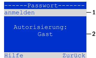
Abbildung 65: An- und Abmeldung
