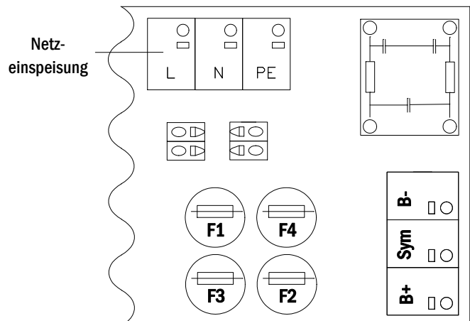
Abbildung 10: Netzeinspeisung
