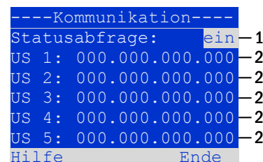
Abbildung 59: IP-Adressen der überwachten Anlagen
