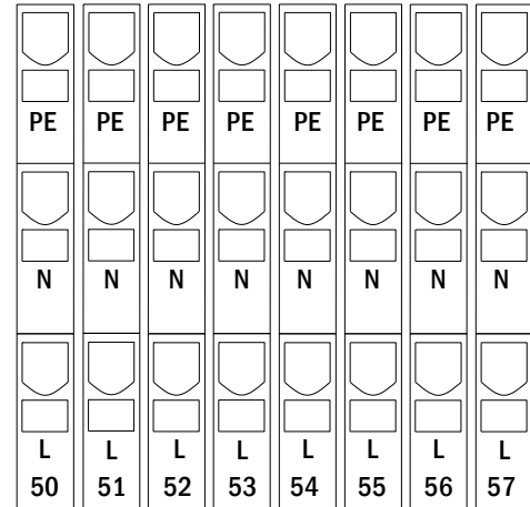
Abbildung 5: SAM-Eingänge
