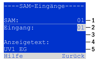
Abbildung 63: Programmierung der SAM-Eingänge
