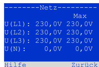
Abbildung 43: Zustand der Netzversorgung
