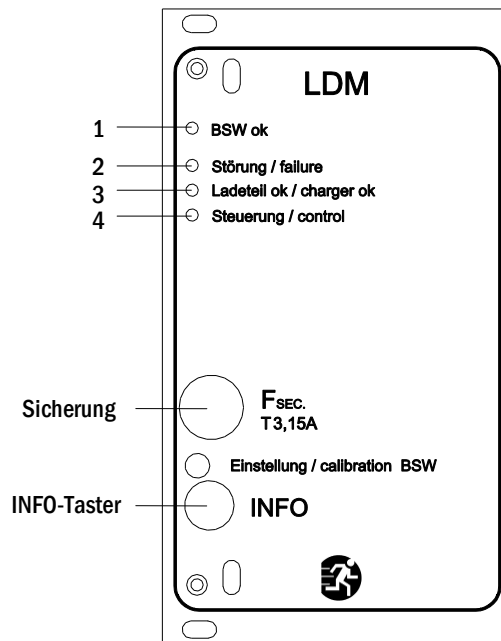
Abbildung 17: Lademodul LDM25
