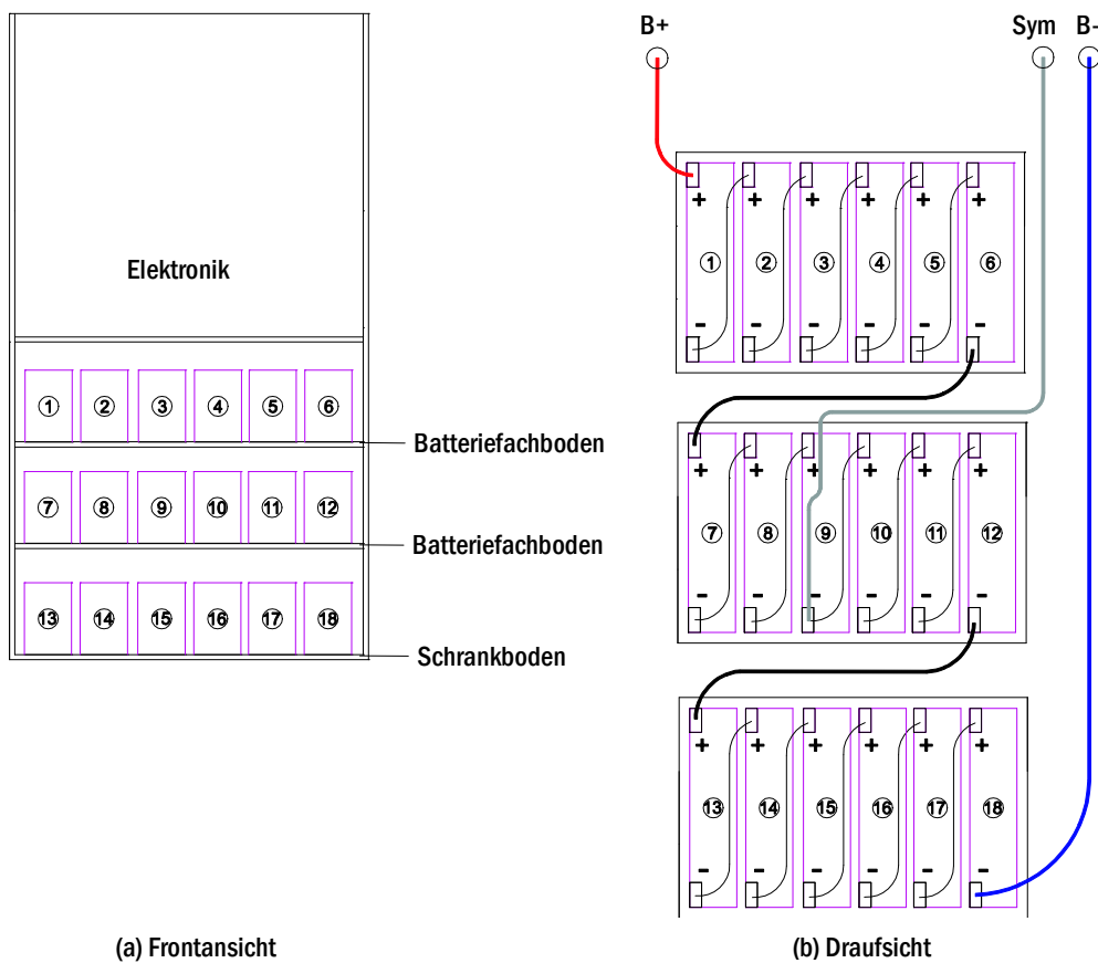
Abbildung 13: Aufstellung und Verschaltung der Batterieblöcke 12V 4,5Ah
