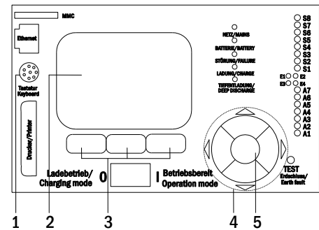
Abbildung 18: Bedienelemente
