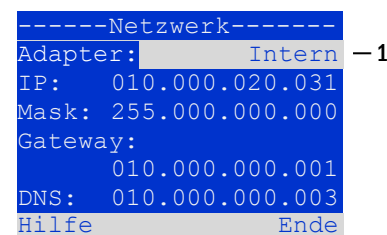
Abbildung 58: Untermenü zum Einrichten der IP-Adressen
