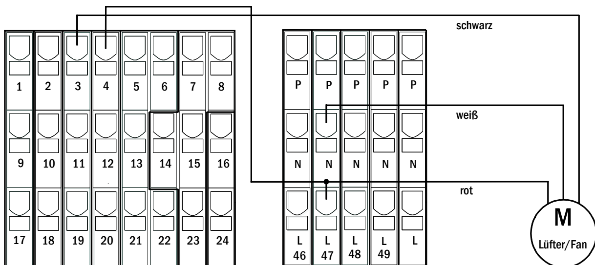
Abbildung 12: Klemmen zum Anschluss eines internen Lüfters
