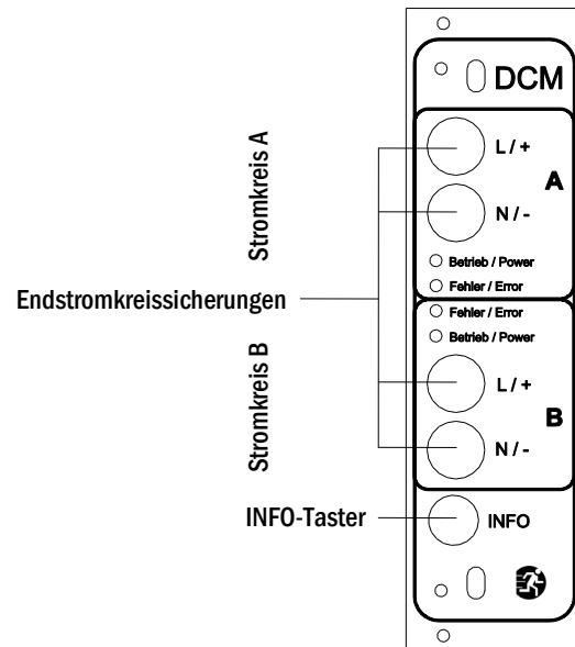
Abbildung 16: DCM-Stromkreismodul
