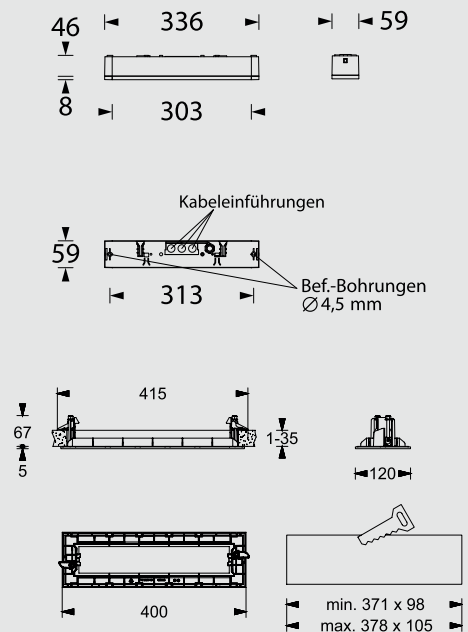
Einbaurahmen
