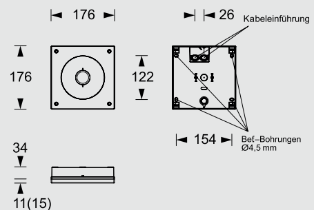
Deckenmontage
