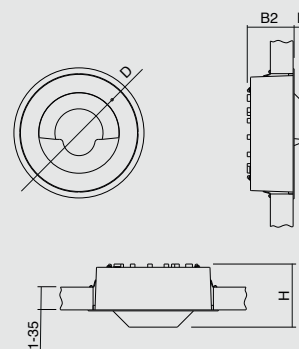
Wandeinbau
